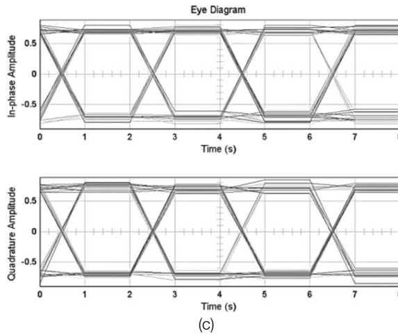
Fig. 13. (a) Diagrama de constelación. (b) Trayectoria de la señal. (c) Diagrama del ojo. Modulación QPSK. Modulación QPSK con E_b/N_0 = 21 .
