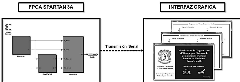
Fig. 14. Diagrama de bloques para la visualización de diagramas en el tiempo a través de la interfaz gráfica.
