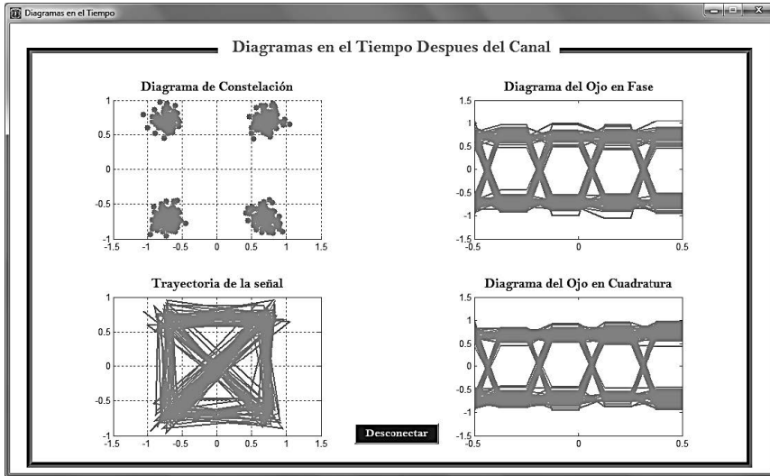
Fig. 16. Diagramas en el tiempo generados por la interfaz gráfica para QPSK con E_b/N_0 = 14 .
