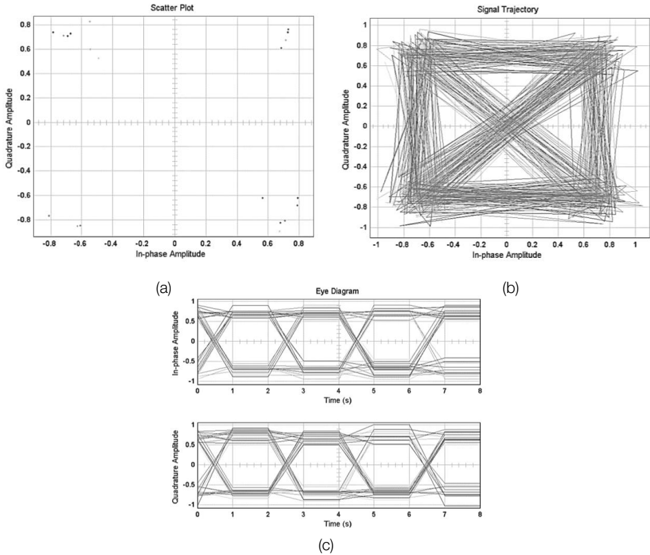
Fig. 12. (a) Diagrama de constelación. (b) Trayectoria de la señal. (c) Diagrama del ojo. Modulación QPSK. Modulación QPSK con E_b/N_0 = 14 .
