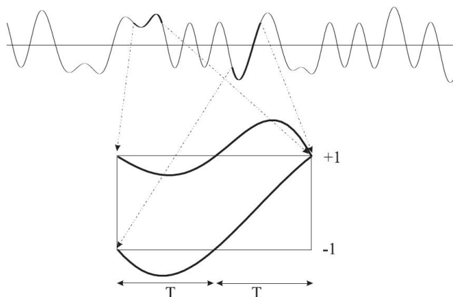
Fig. 3. Proceso de construcción de un diagrama de ojo.
