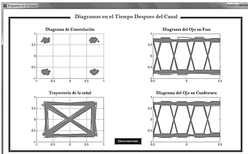
Fig. 17. Diagramas en el tiempo generados por la interfaz gráfica para QPSK con E_b/N_0 = 21 .
