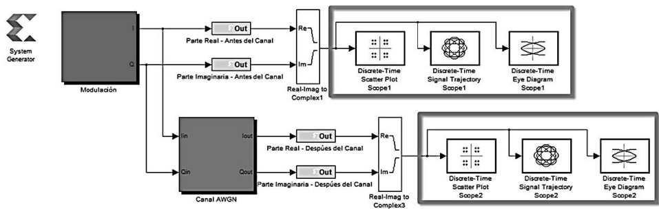
Fig. 10. Bloques de Simulink para graficar diagramas en el tiempo.
