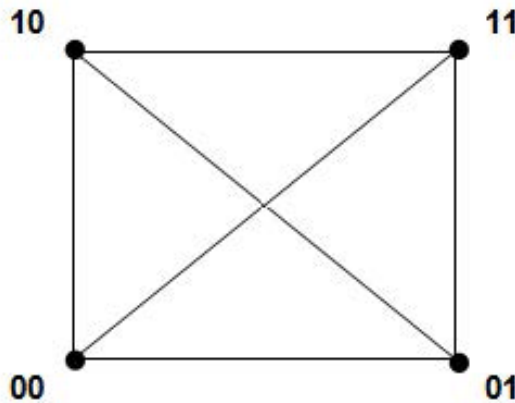
Fig. 2. Trayectoria de la señal para QPSK.
