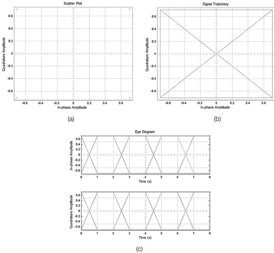
Fig. 11. (a) Diagrama de constelación. (b) Trayectoria de la señal. (c) Diagrama del ojo. Modulación QPSK.
