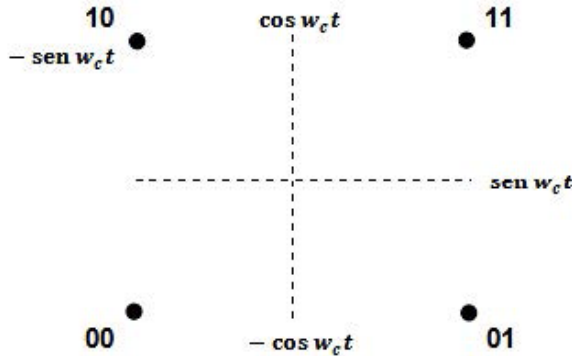
Figura 1. Diagrama de constelación para QPSK.
