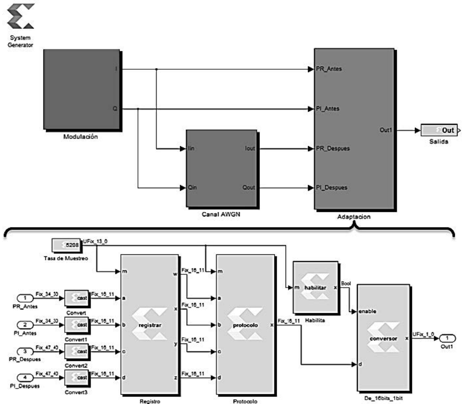
Fig. 5. Modelo en Simulink con SysGen para la adaptación de los datos.
