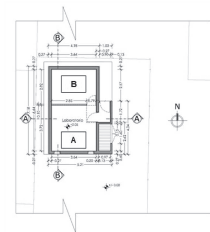
Figura 5. Planta General del LEVS. Figura 6. Envoltante del LEVS.
