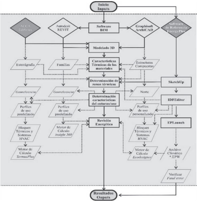
Figura 7. Mecánica de Trabajo para pasar de un modelo BIM a un modelo BEM
