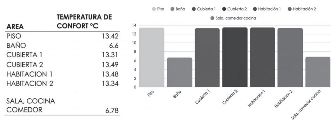
Gráfico 4. Temperatura de Confort en °C en ladrillos de hormigón. Nota. Elaboración por autores, 2025.
