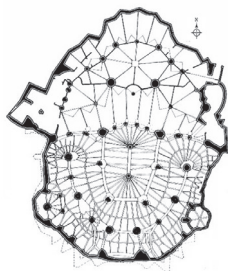
Figura 21. Cripta de la Colonia Güell, Santa Coloma de Cervelló (Cataluña), planta.
