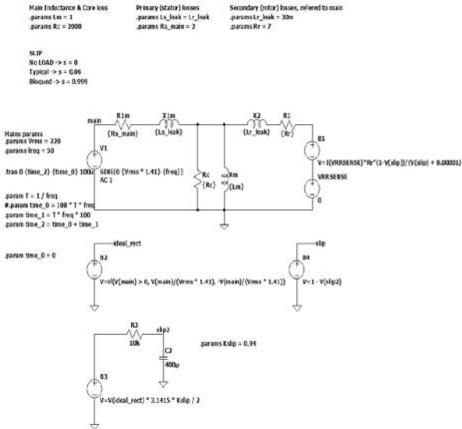
Figura 7: circuito utilizado para la simulación del comportamiento dinámico.
